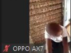
Android Bluedroid4...
